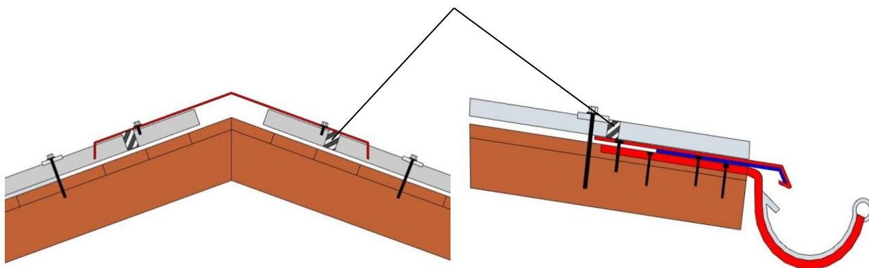
Umístění těsnění
