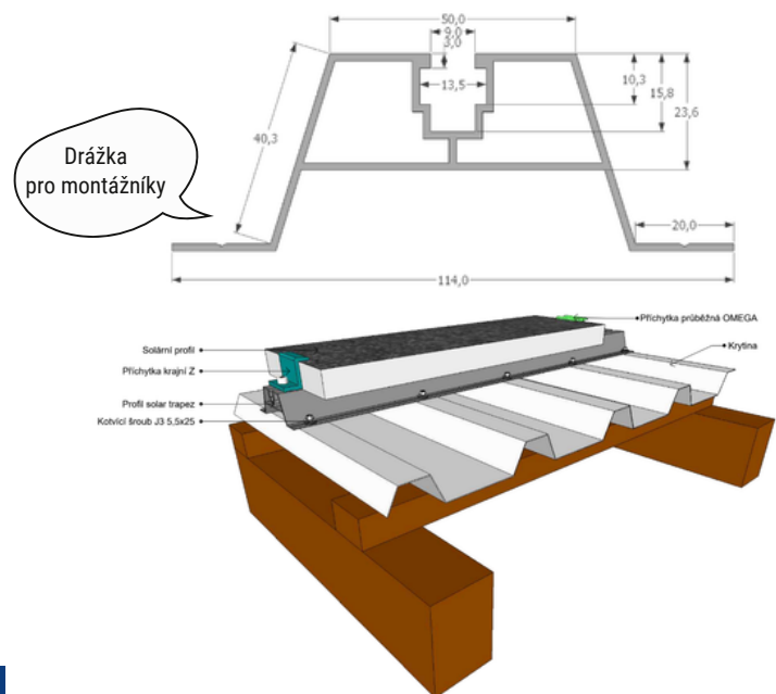
Sestava spoje mezi panely
