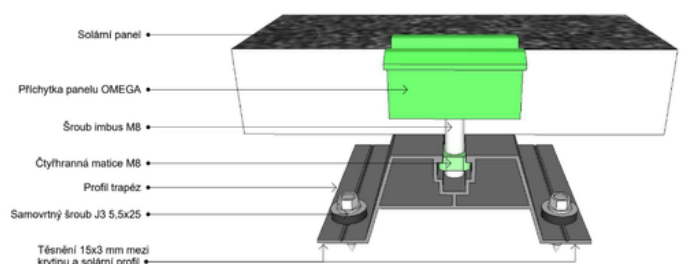
Sestava spoje mezi panely
