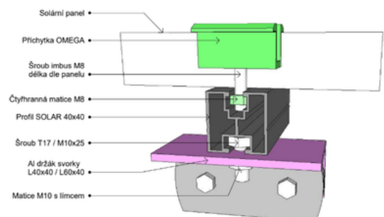
Sestava spoje mezi panely
